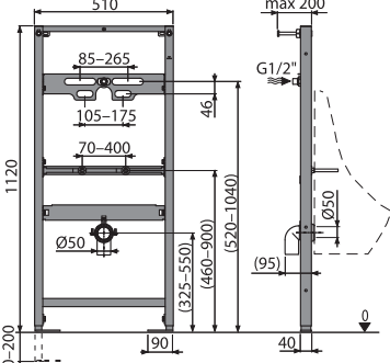
A107/1120 Монтажная рама для писсуара
