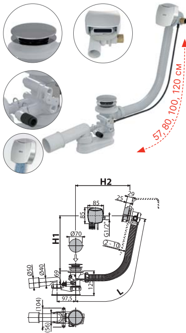
A566-273133-57 Сифон для гидромассажных ванн с напуском через перелив, металл
