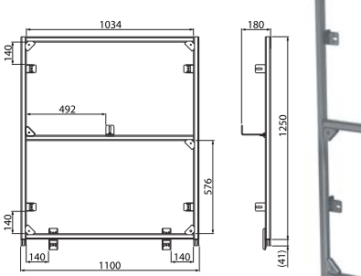
AS101-SET02, AS101-SET02-PR * Системная стена
