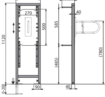
A106/1120 Монтажная рама для поручней
