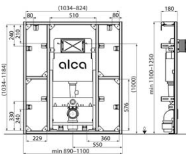
AS101-SET01, AS101-SET01-PR * Системная стена + Скрытая система инсталляции
