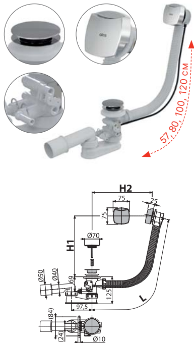
A566-112122-57 Сифон для гидромассажных ванн, хром
