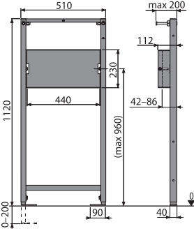
A104PB/1120 Монтажная рама для смесителя скрытого монтажа
