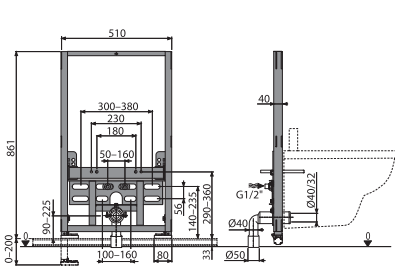
AS105/850 Монтажная рама для биде
