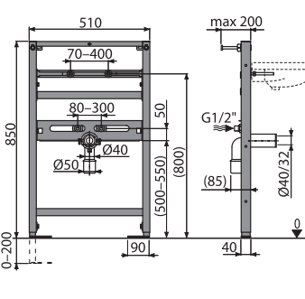
A104/850 Монтажная рама для умывальника
